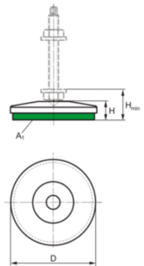
Croquis de montage
