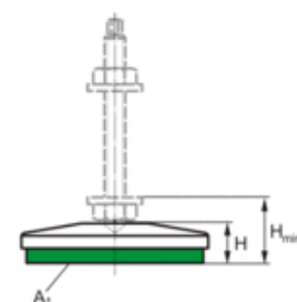
Massskizze
