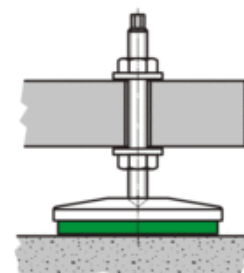
Einbauskizze
