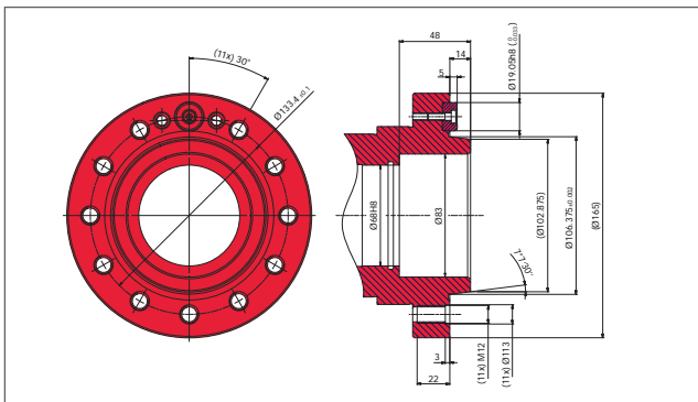
Nez de broche A2-6 Spindelhase A2-6 Spindle nose A2-6
