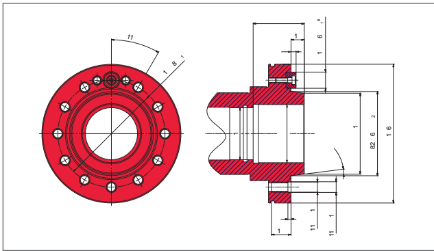
Nez de broche A2-5 Spindelhase A2-5 Spindle nose A2-5
